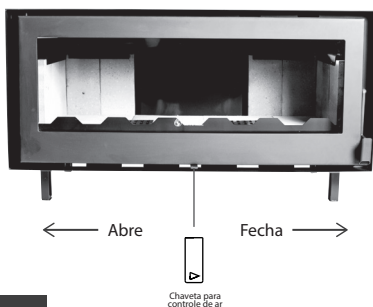
ESQUEMA LAREIRAS LINHA ABRUZZO / NOVARA / TOSCANA
